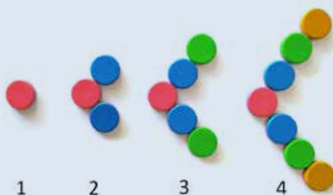
Figure 14. Aspect procédural.
